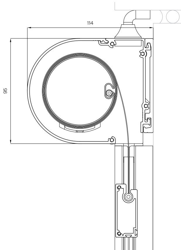
Vertikalsnitt av D-formad kasett med bottenprofil, 1:2
