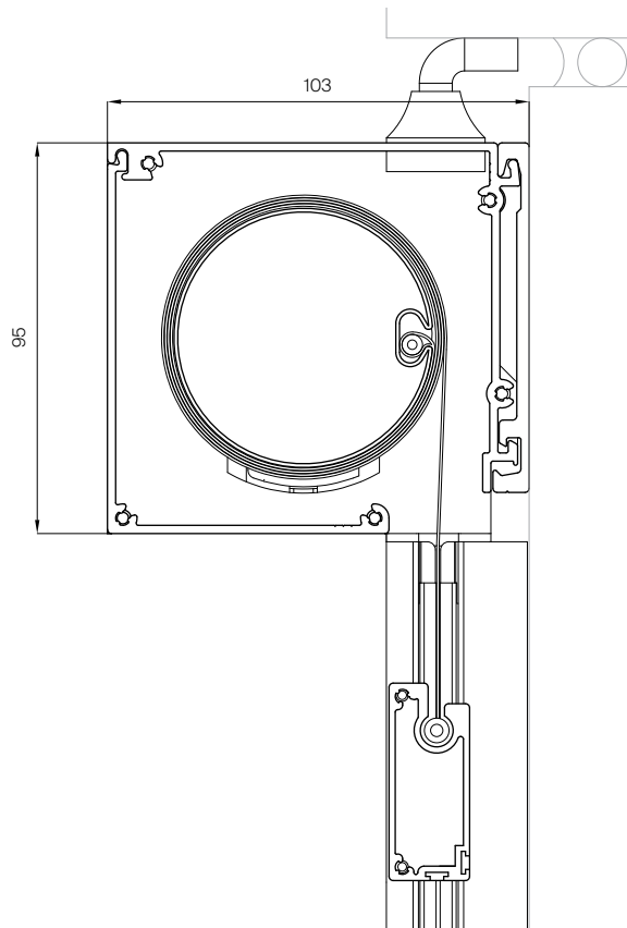
Vertikalsnitt av fyrkantig kasett med bottenprofil, 1:2
