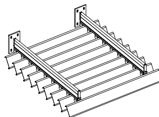
Skærm med for- og sidekant
