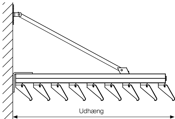
Lodret snit af horisontal skærm uden forkant
