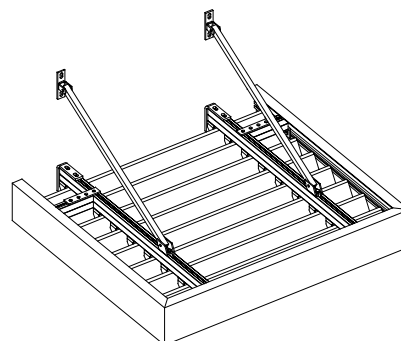
Skærm med for- og sidekant
