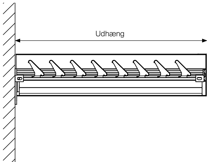
Lodret snit af horisontal skærm uden forkant
