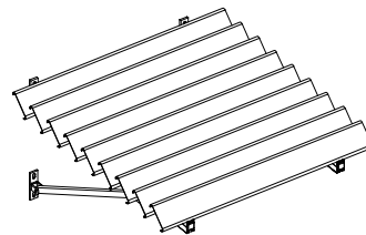
Skærm med for- og sidekant
