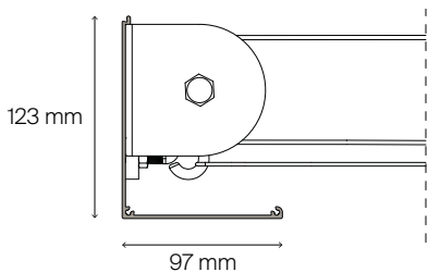
Afdækningsprofil i side med hjulbe- slag, motorplacering 'A'
