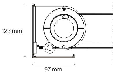
Afdækningsprofil i side med motorbe- slag, motorplacering 'B'
