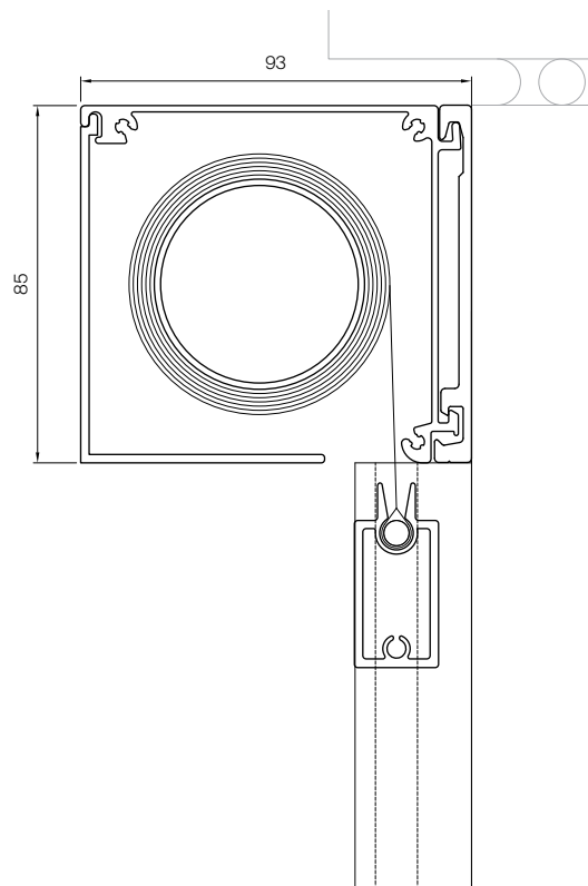
Vertikalsnitt av fyrkantig kasett med bottenprofil, 1:2
