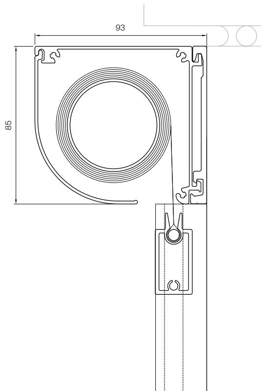
Vertikalsnitt av rundad kasett med bottenprofil, 1:2
