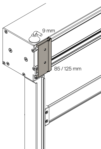
Vægmonteret
