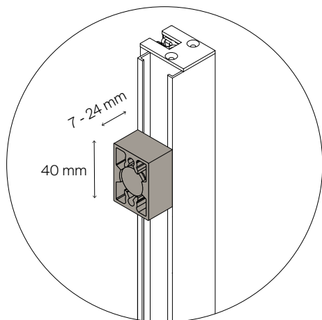
<25 mm distancestykke
