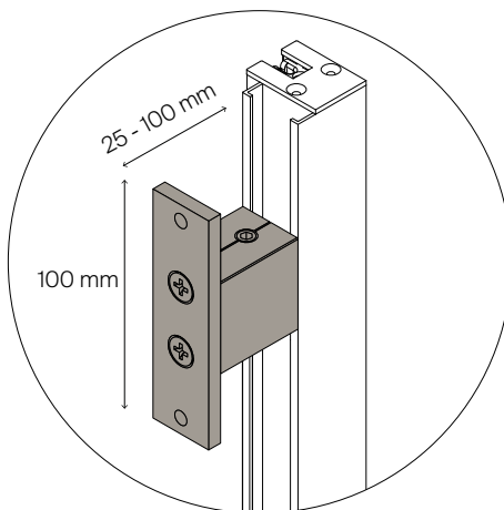
≥25 mm distancestykker
