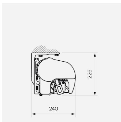
Takmontering
