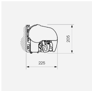
Väggmontering
