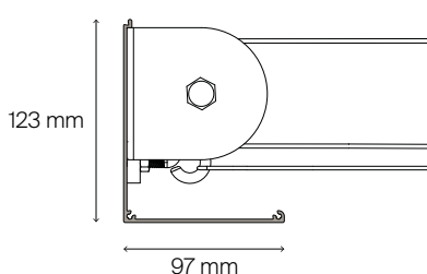
Profil för sidokåpa med hjulhus, motorplacering 'A'
