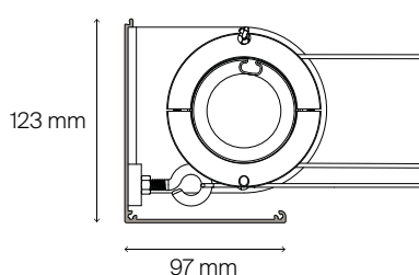
Profil för sidokåpa med motorfäste, motorplacering 'B'
