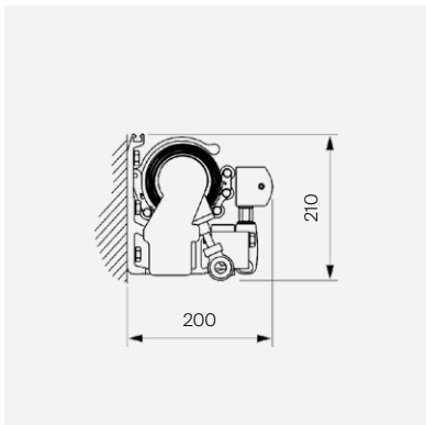
Väggmontering
