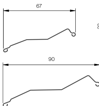
Vertical sektion lamell 1:2
