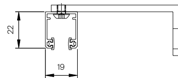
Horizontalsnitt sidofält 1:2
