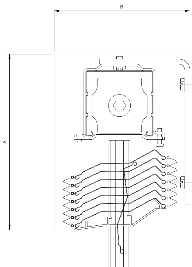
Vertical sektion 1:2
