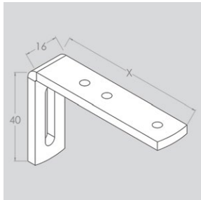
Vinkel til vægmontering X = 3, 5, 7, 9, 12, 14, 16, 20 \text{ cm}
