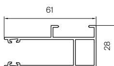
Vandret snit af sideliste
