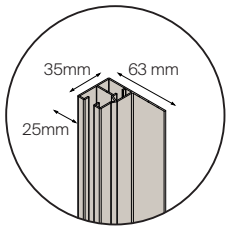
Niche sideprofil
