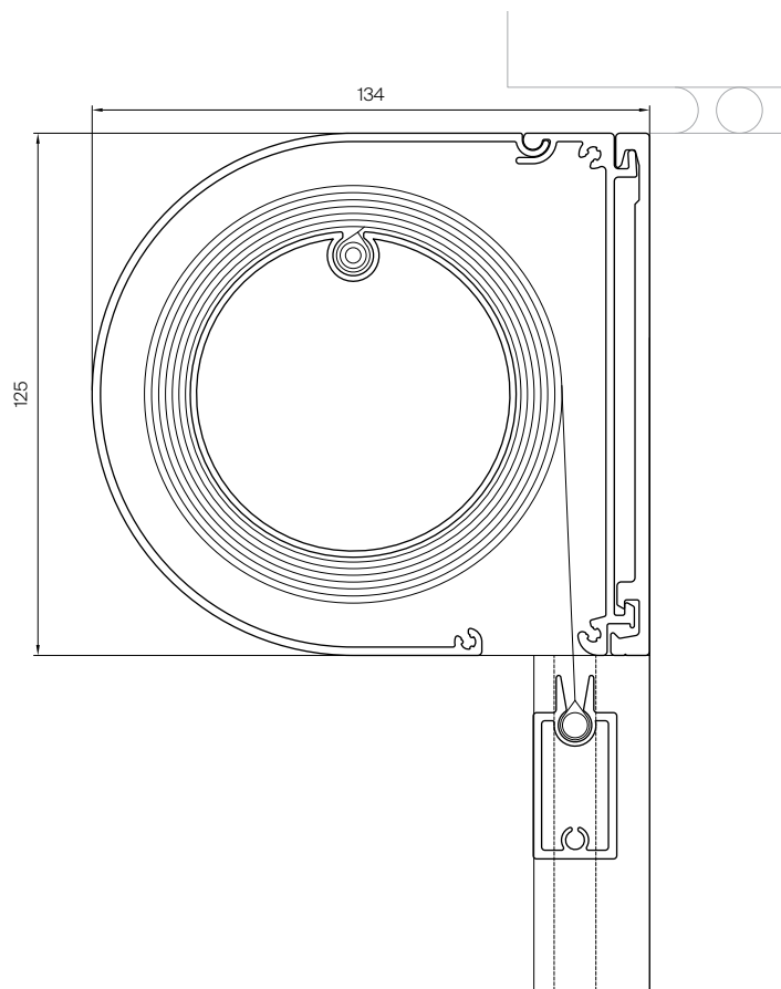
Lodret snit af D-formet kasse med bundprofil, 1:2
