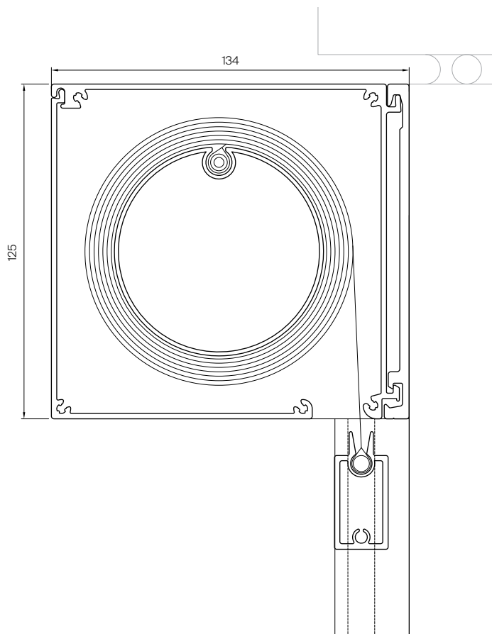
Lodret snit af firkantet kasse med bundprofil, 1:2
