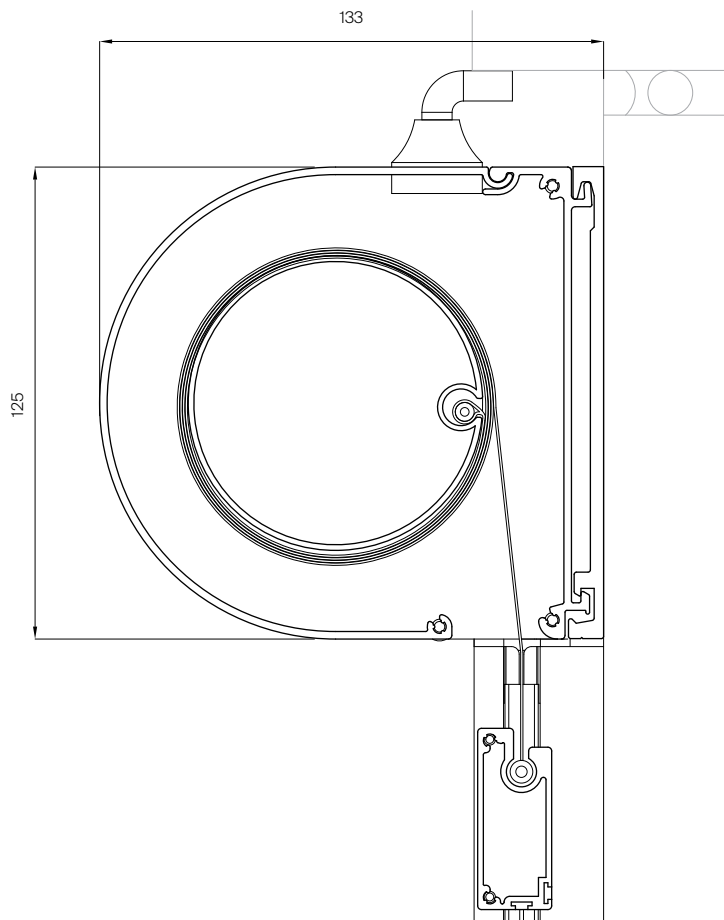
Vertikalsnitt av D-formad kasett med bottenprofil, 1:2
