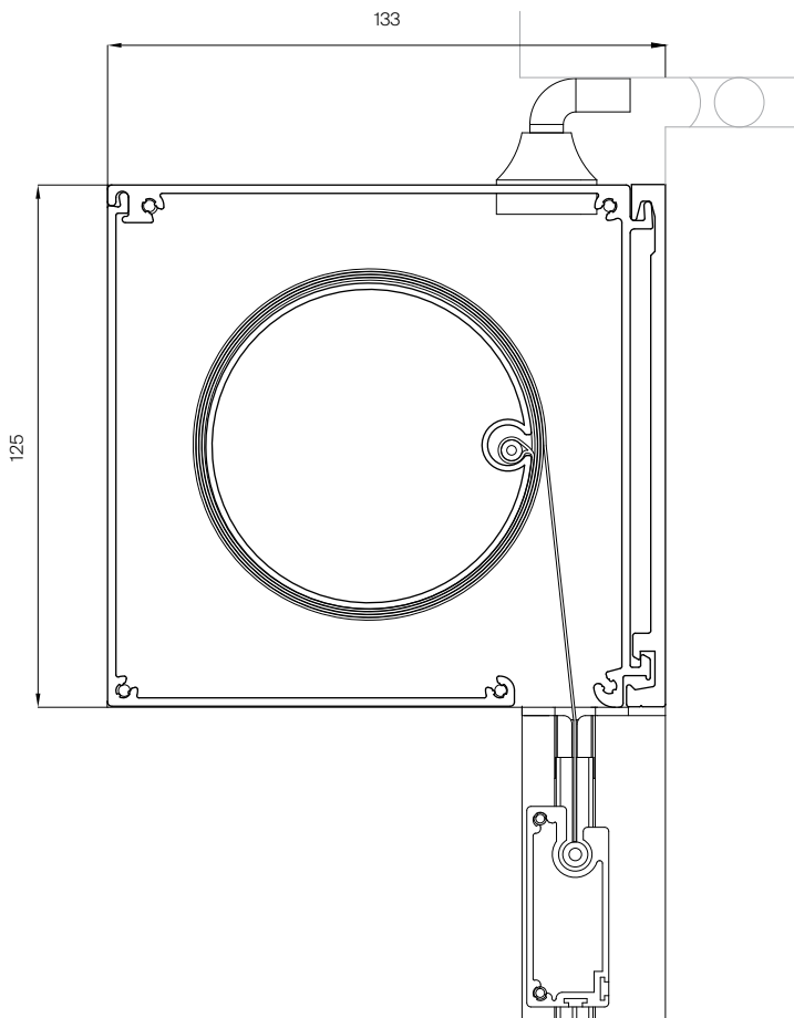
Vertikalsnitt av fyrkantig kasett med bottenprofil, 1:2
