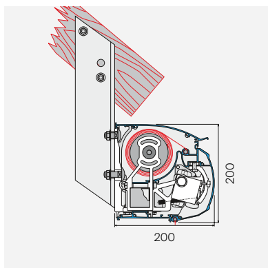
Spærmontage lodret
