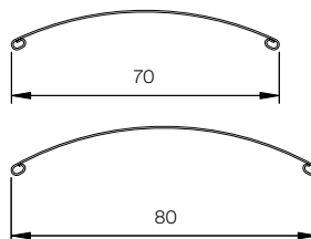
Vertical sektion lamell 1:2
