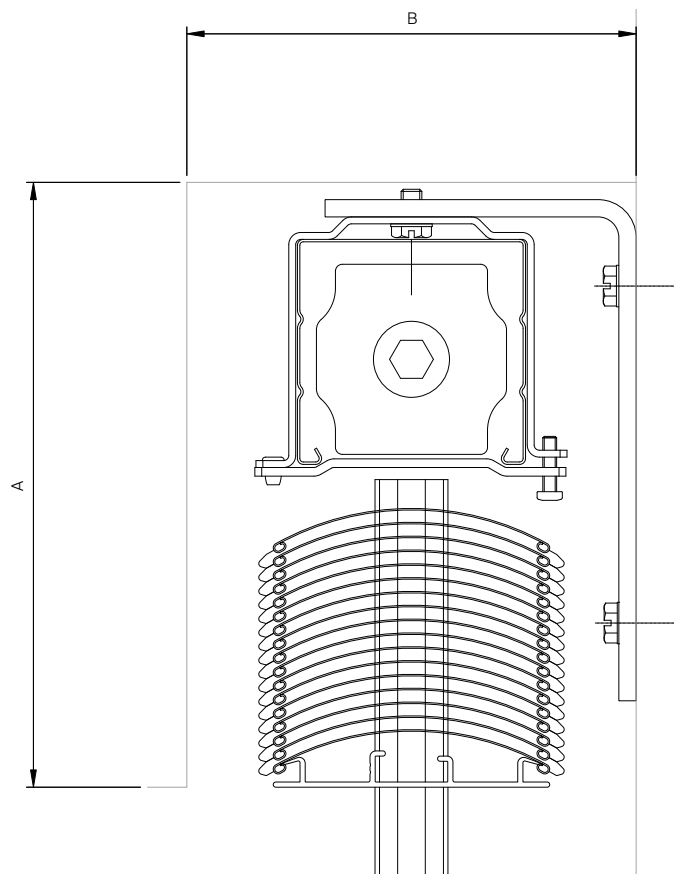
Vertical sektion 1:2
