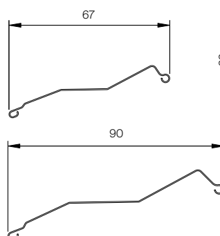
Lodret snit lamel 1:2
