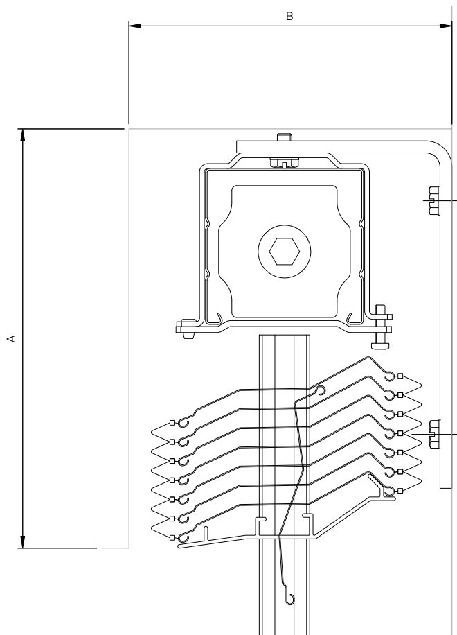
Lodret snit 1:2
