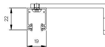
Vandret snit sideliste 1:2
