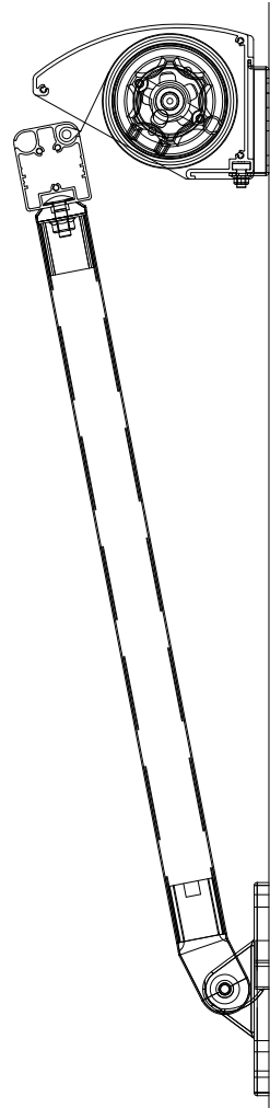
Modell med vridstång/motor (stora armar/stort frontprofil)
