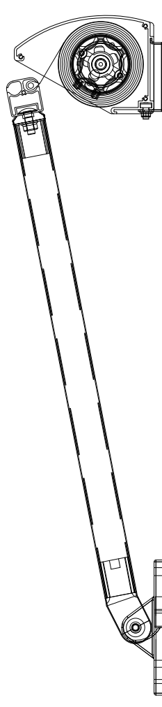
Modell med vridstång/motor (stora armar)
